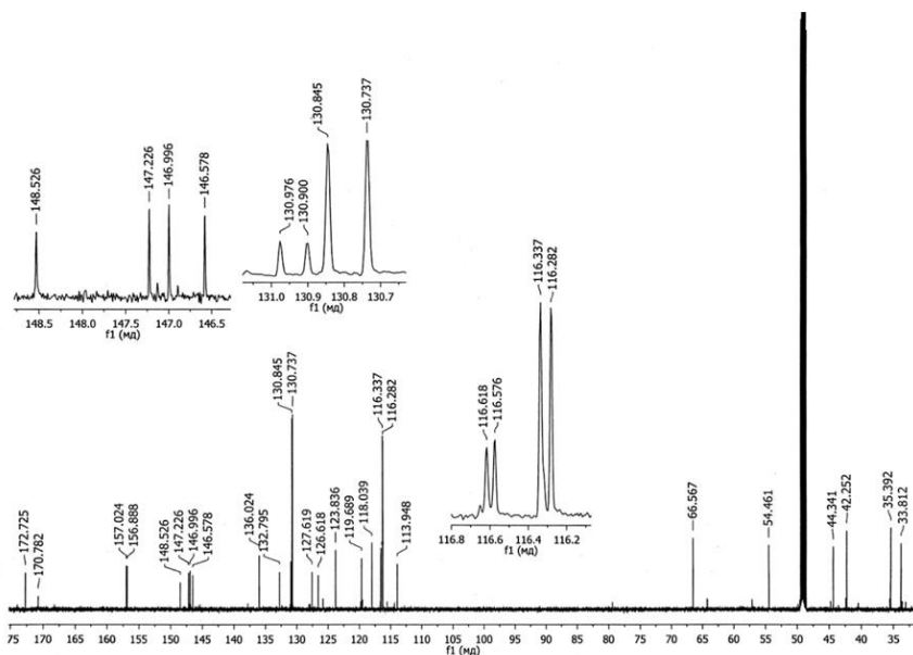
3-rasm. Tadqiq qilinayotgan moddaning uglerod va vodorod atomlari yadrolari orasidagi spin-spin o'zaro ta'sir to'liq so'ndirib olingan ^{13}\text{C} YaMR spektri
