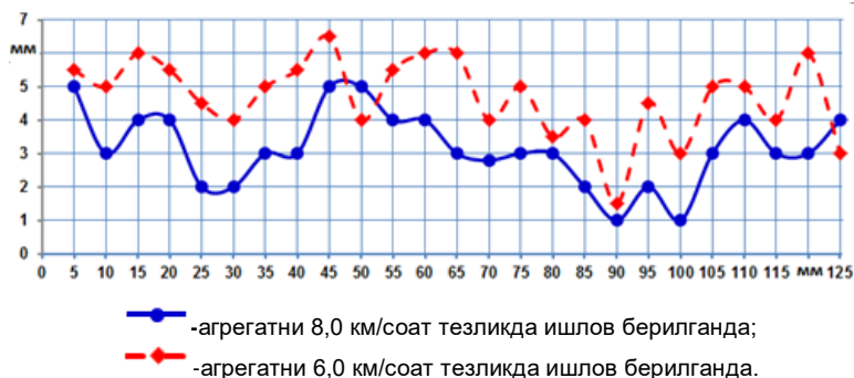
2-расм. Чизел юмшаткич билан ишлов берилган даланинг кўндаланг профили
